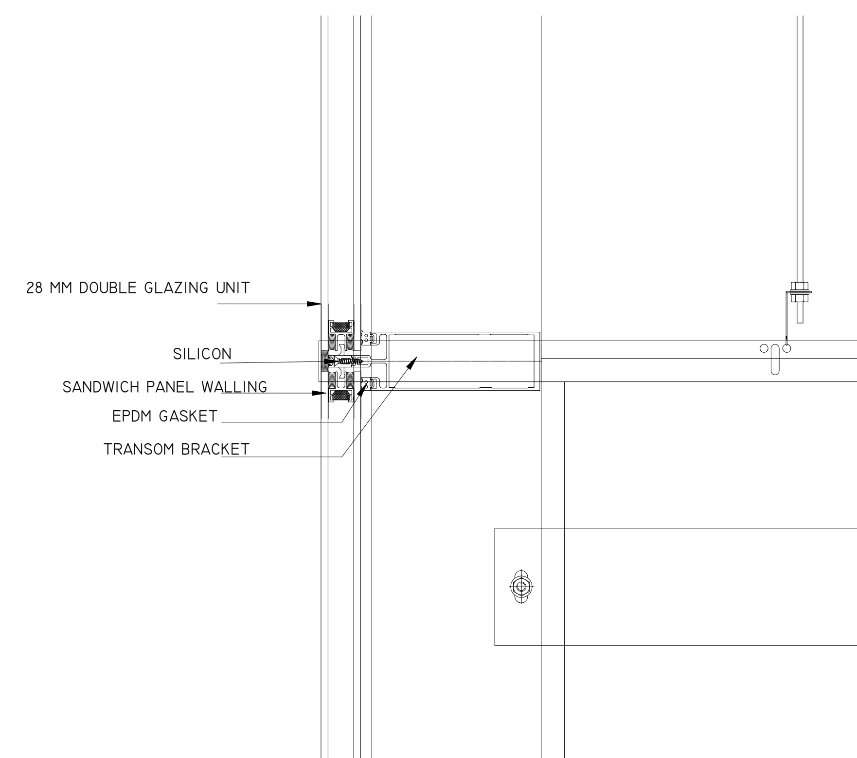
6 CURTAIN WALL CONNECTION 1 : 5
